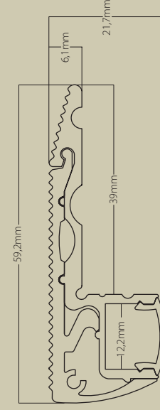
Star 22 Multilínea Multiline
