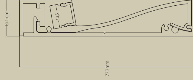
Star 29 Zócalo Baseboard
