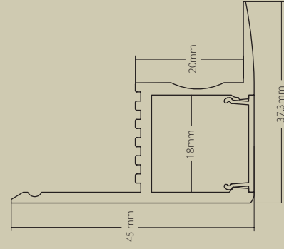
Star 11 Pladur Plasterboard
