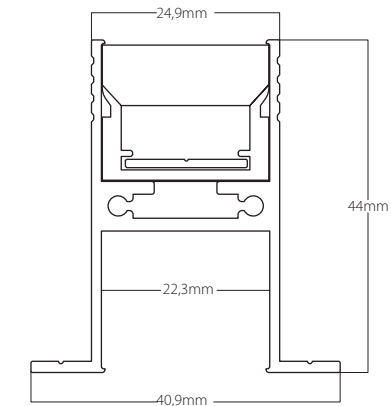
233015070 Perfil aluminio polivalente para preinstalación, superficie o empotrado Polyvalent aluminium profile for pre-installation, surface or recessed
