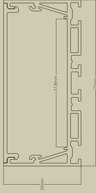
Star 23 Cornisa Cornice
